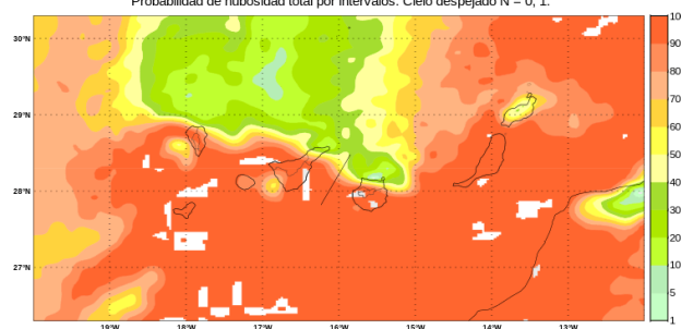
ENS-IFS (0.1°) 20260809 a 00 UTC. H+090. Validez: miércoles, 12 de agosto de 2026, a 18 UTC. Probabilidad de nubosidad total por intervalos. Cielo despejado N = 0, 1.
