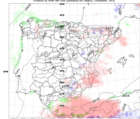
CTRL-IFS (0.1°) 20260809 a 00 UTC. H+090. Validez: miércoles, 12 de agosto de 2026, a 18 UTC. Nubosidad compuesta. Nubes bajas en verde, nubes medias en azul y nubes altas en rosa. Presión al nivel del mar (isobaras en negro). Unidades: hPa.
