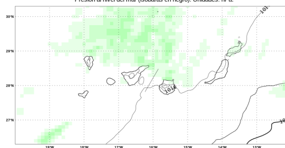
CTRL-IFS (0.1°) 20260809 a 00 UTC. H+090. Validez: miércoles, 12 de agosto de 2026, a 18 UTC. Nubosidad compuesta. Nubes bajas en verde, nubes medias en azul y nubes altas en rosa. Presión al nivel del mar (isobaras en negro). Unidades: hPa.
