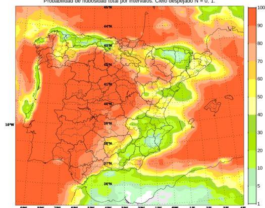
ENS-IFS (0.1°) 20260809 a 00 UTC. H+090. Validez: miércoles, 12 de agosto de 2026, a 18 UTC. Probabilidad de nubosidad total por intervalos. Cielo despejado N = 0, 1.
