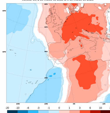
Anomalia de temperatura a 2 m. Unidades: °C. Validez: del 2 de marzo de 2026 al 8 de marzo de 2026.
