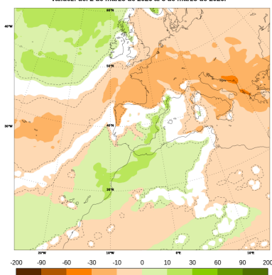
Anomalia de precipitación acumulada. Unidades: mm. Validez: del 2 de marzo de 2026 al 8 de marzo de 2026.
