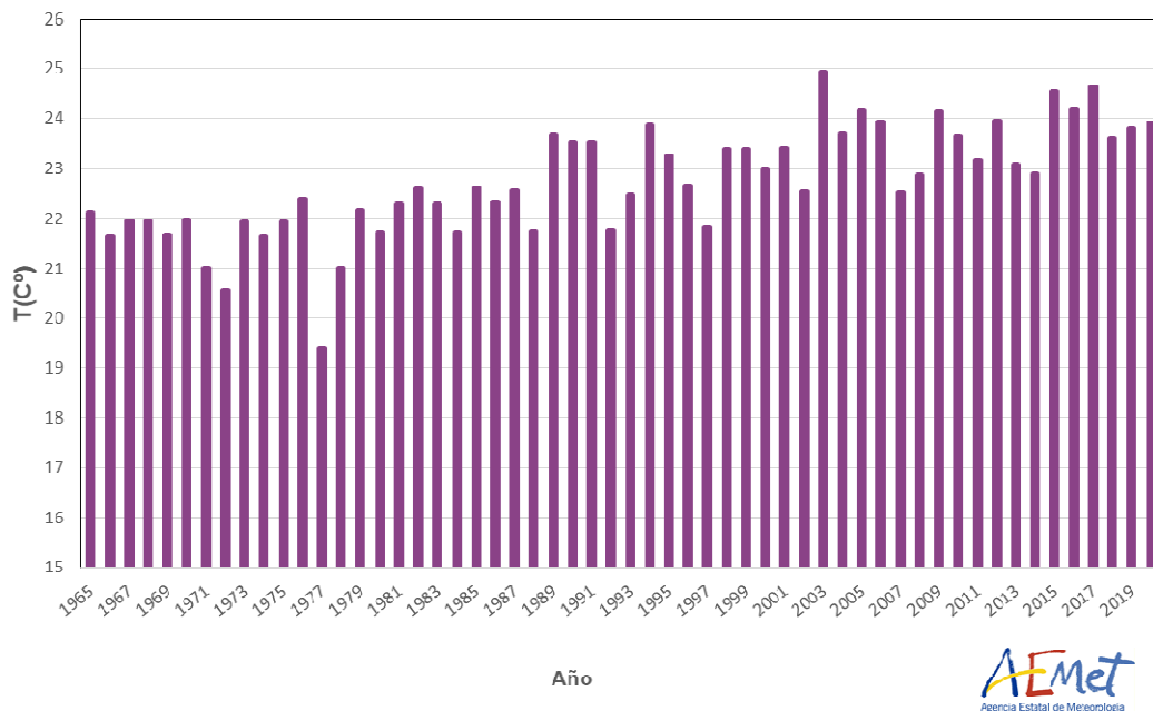
Serie de temperaturas medias en España en el trimestre junio-julio-agosto (1965-2020)
