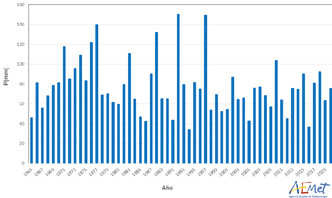
Serie de precipitaciones medias sobre España en el trimestre junio-julio-agosto (1965-2020)
