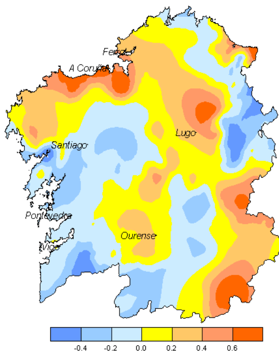
Fig. 1. Anomalías de temperatura. (°C de diferencia con el valor normal 1981-2010).
