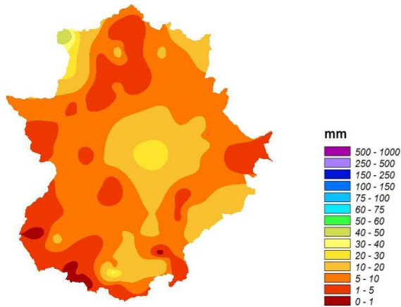
Precipitación Mensual Junio de 2025
