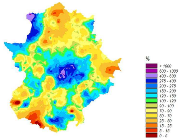
Porcentaje sobre Precipitación Mensual Junio de 2025
