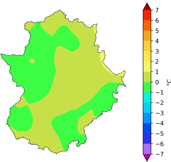
Anomalía de temperatura media
