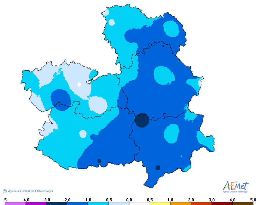
enero 2017: Anomalía de la temperatura media mensual respecto al periodo 1981-2010
