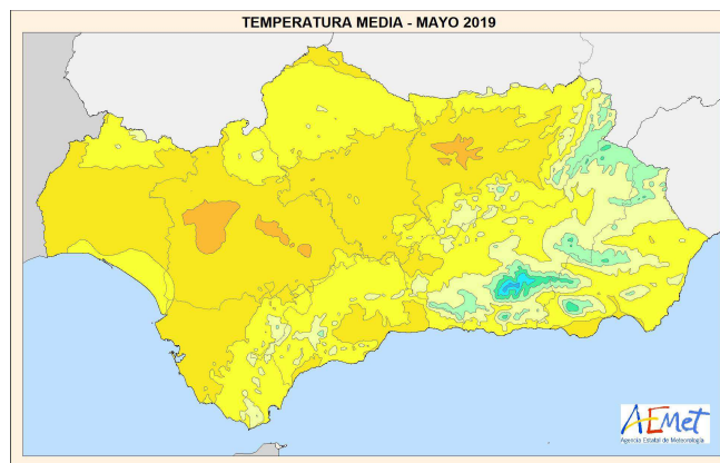
Temperatura media
