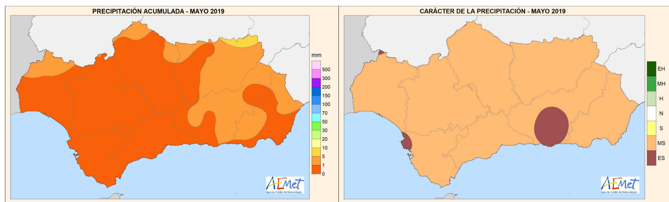
Precipitación mensual
