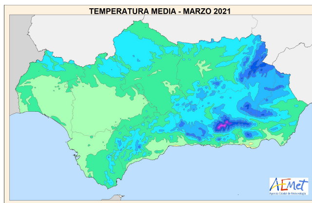
Temperatura media
