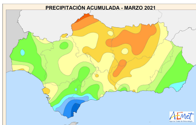
Precipitación mensual
