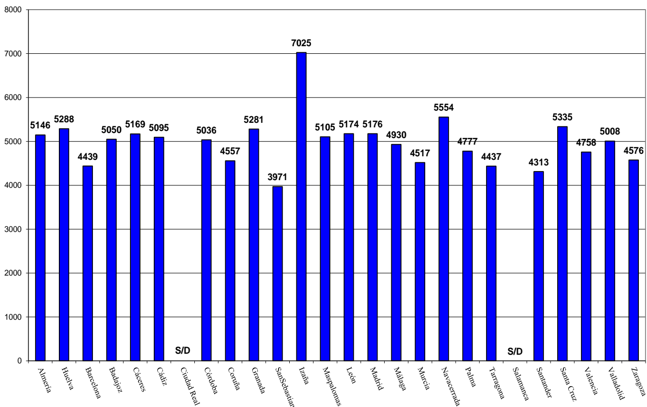
VALORES MEDIO DIARIOS DE RADIACIÓN UV Eritemática EN DISTINTAS ESTACIONES DE LA RED JULIO/2022(J/m 2 )
