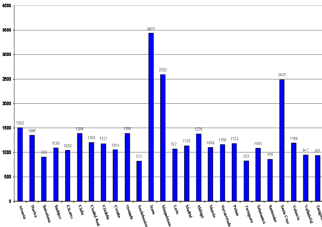
VALORES MEDIO DIARIOS DE RADIACIÓN UV Eritemática EN DISTINTAS ESTACIONES DE LA RED FEBRERO/2021(J/m 2 )
