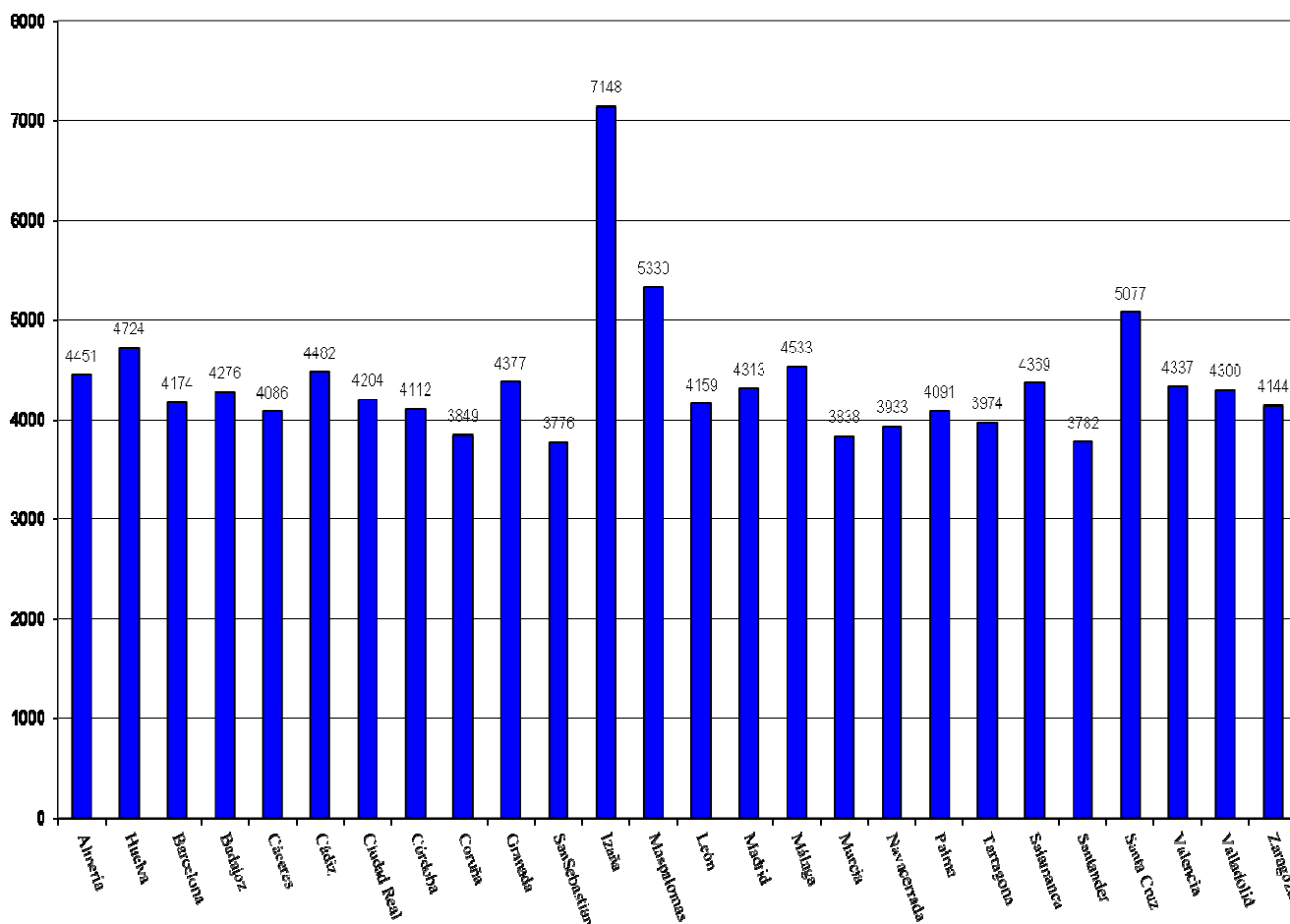
VALORES MEDIO DIARIOS DE RADIACIÓN UV Eritemática EN DISTINTAS ESTACIONES DE LA RED MAYO/2020(J/m 2 )
