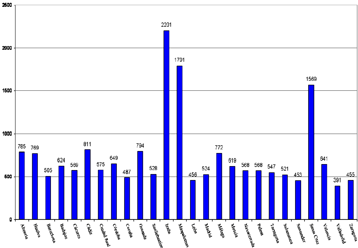
VALORES MEDIO DIARIOS DE RADIACIÓN UV Eritemática EN DISTINTAS ESTACIONES DE LA RED ENERO/2020(J/m 2 )
