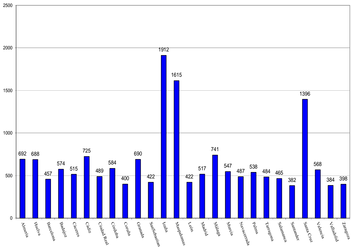
VALORES MEDIO DIARIOS DE RADIACIÓN UV Eritemática EN DISTINTAS ESTACIONES DE LA RED DICIEMBRE/2019(J/m 2 )
