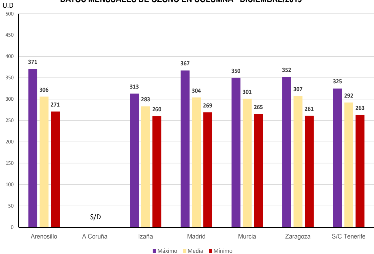
DATOS MENSUALES DE OZONO EN COLUMNA - DICIEMBRE/2019
