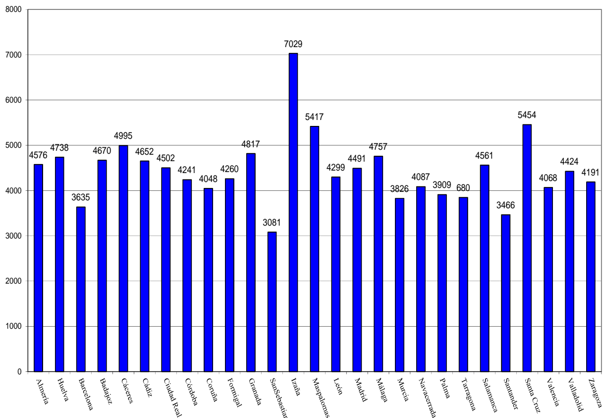
VALORES MEDIO DIARIOS DE RADIACIÓN UV Eritemática EN DISTINTAS ESTACIONES DE LA RED MAYO/2019(J/m 2 )
