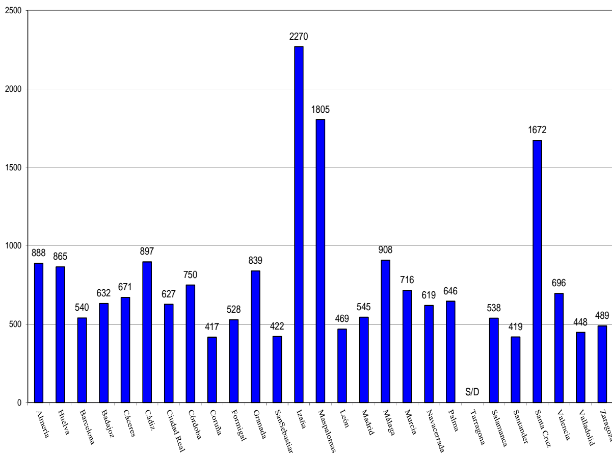
VALORES MEDIO DIARIOS DE RADIACIÓN UV Eritemática EN DISTINTAS ESTACIONES DE LA RED DICIEMBRE/2018(J/m 2 )
