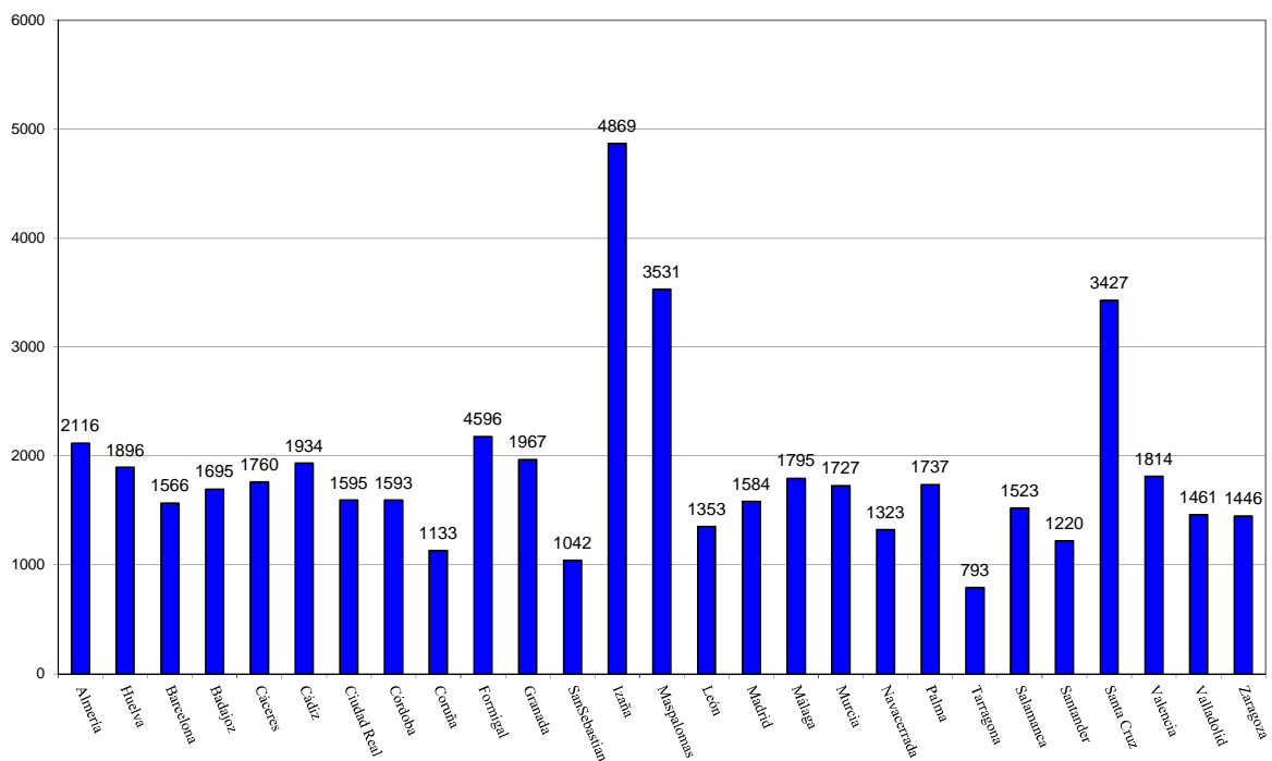
VALORES MEDIO DIARIOS DE RADIACIÓN UV Eritemática EN DISTINTAS ESTACIONES DE LA RED MARZO/2018(J/m 2 )
