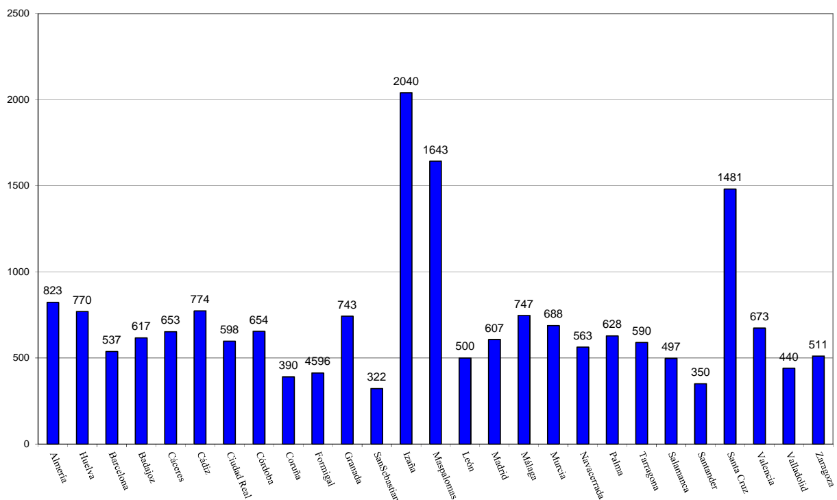
VALORES MEDIO DIARIOS DE RADIACIÓN UV Eritemática EN DISTINTAS ESTACIONES DE LA RED Enero/2018(J/m 2 )
