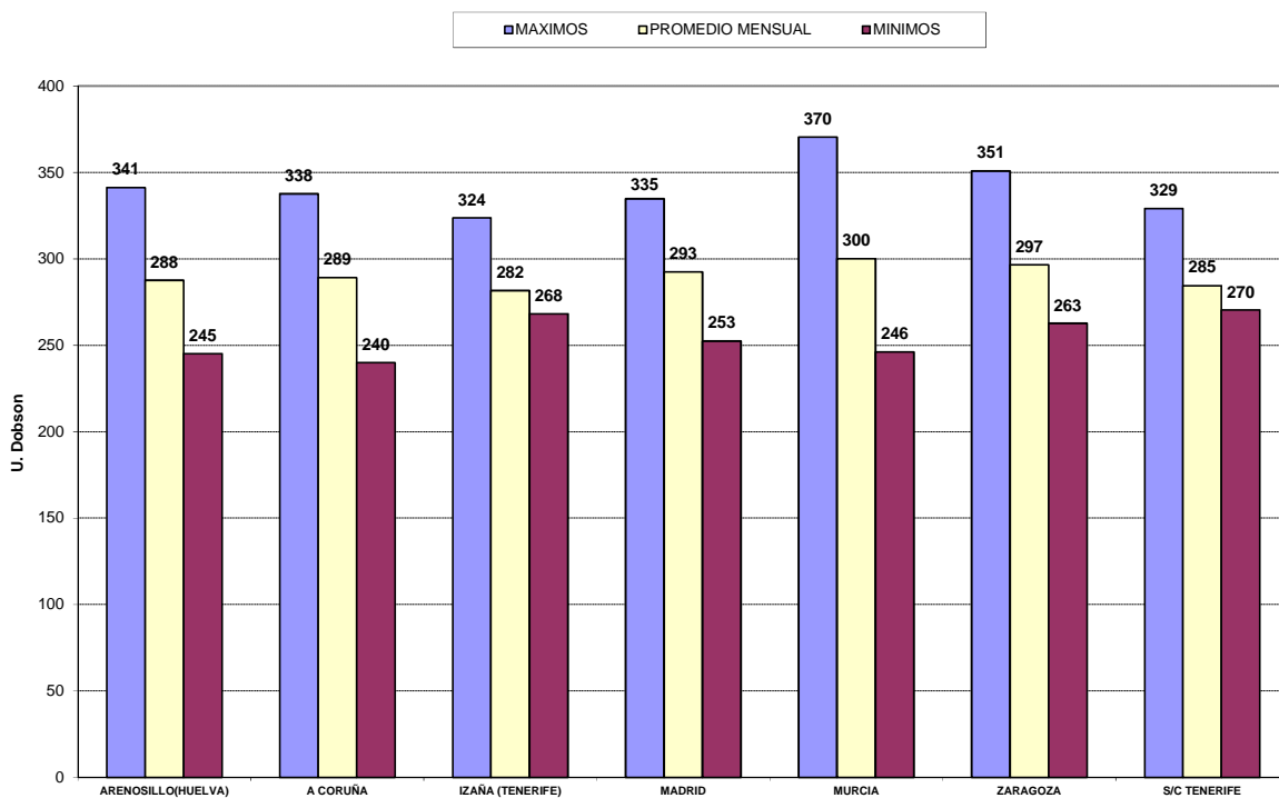
DATOS MENSUALES DE OZONO EN COLUMNA - DICIEMBRE 2017
