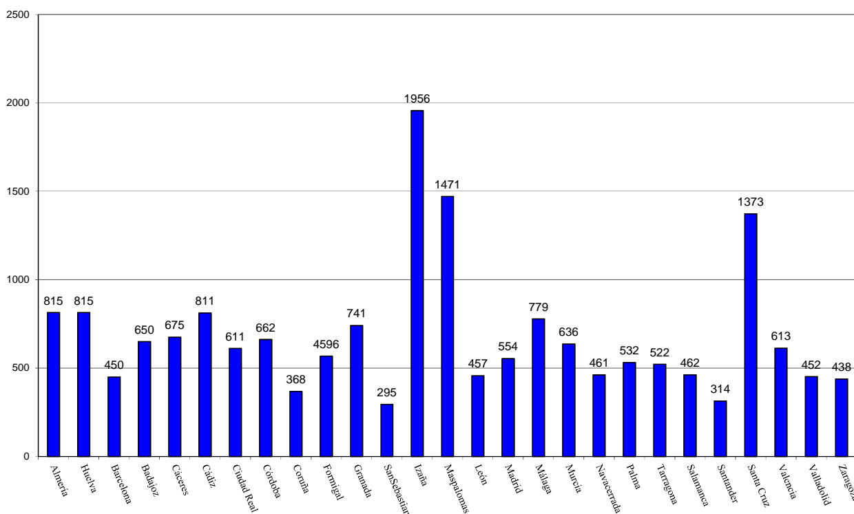
VALORES MEDIO DIARIOS DE RADIACIÓN UV Eritemática EN DISTINTAS ESTACIONES DE LA RED DICIEMBRE/2017 (J/m 2 )
