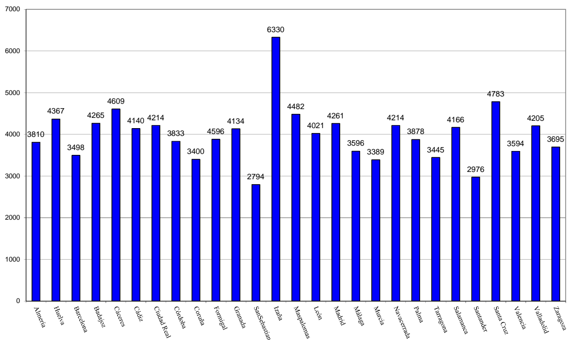
VALORES MEDIO DIARIOS DE RADIACIÓN UV Eritemática EN DISTINTAS ESTACIONES DE LA RED AGOSTO/2017 (J/m 2 )
