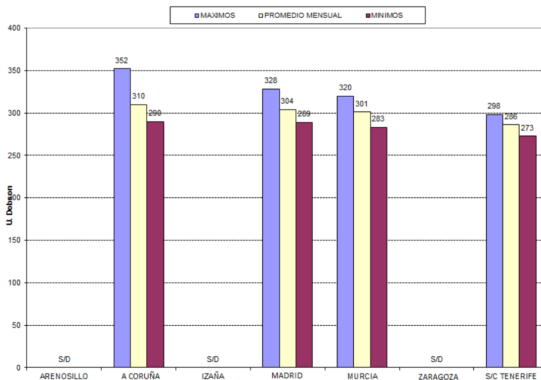
DATOS MENSUALES DE OZONO EN COLUMNA - AGOSTO 2017
