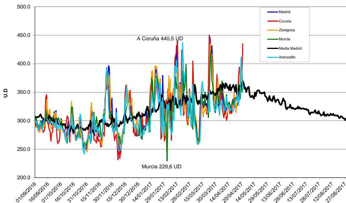
OZONO TOTAL EN COLUMNA - AÑO AGRÍCOLA 2016-2017
