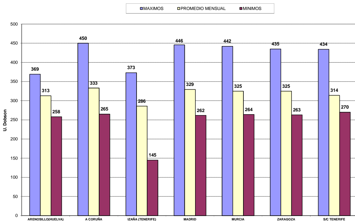
DATOS MENSUALES DE OZONO EN COLUMNA - ABRIL 2017
