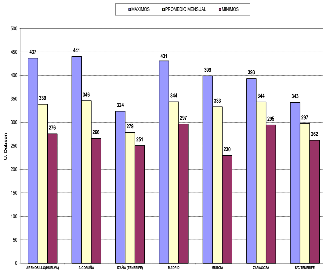
DATOS MENSUALES DE OZONO EN COLUMNA - FEBRERO 2017
