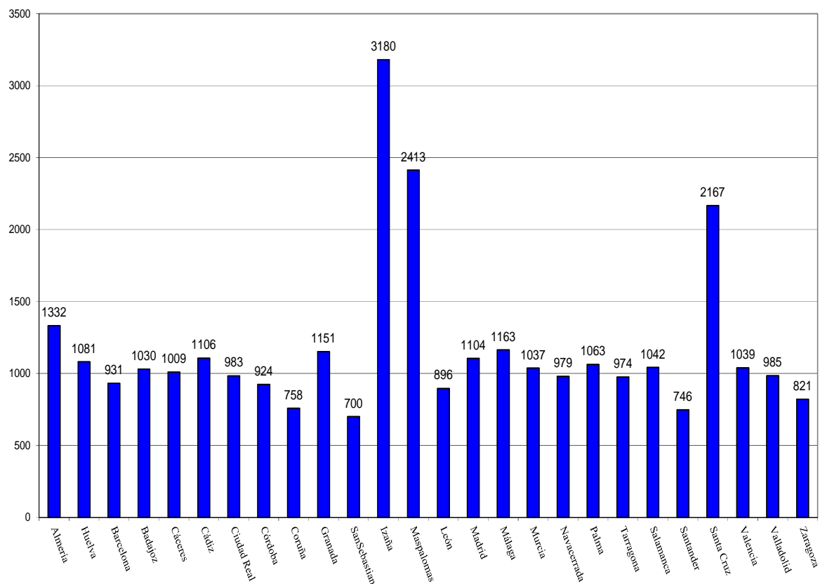
VALORES MEDIO DIARIOS DE RADIACIÓN UV Eritemática EN DISTINTAS ESTACIONES DE LA RED FEBRERO-2017 (J/m 2 )
