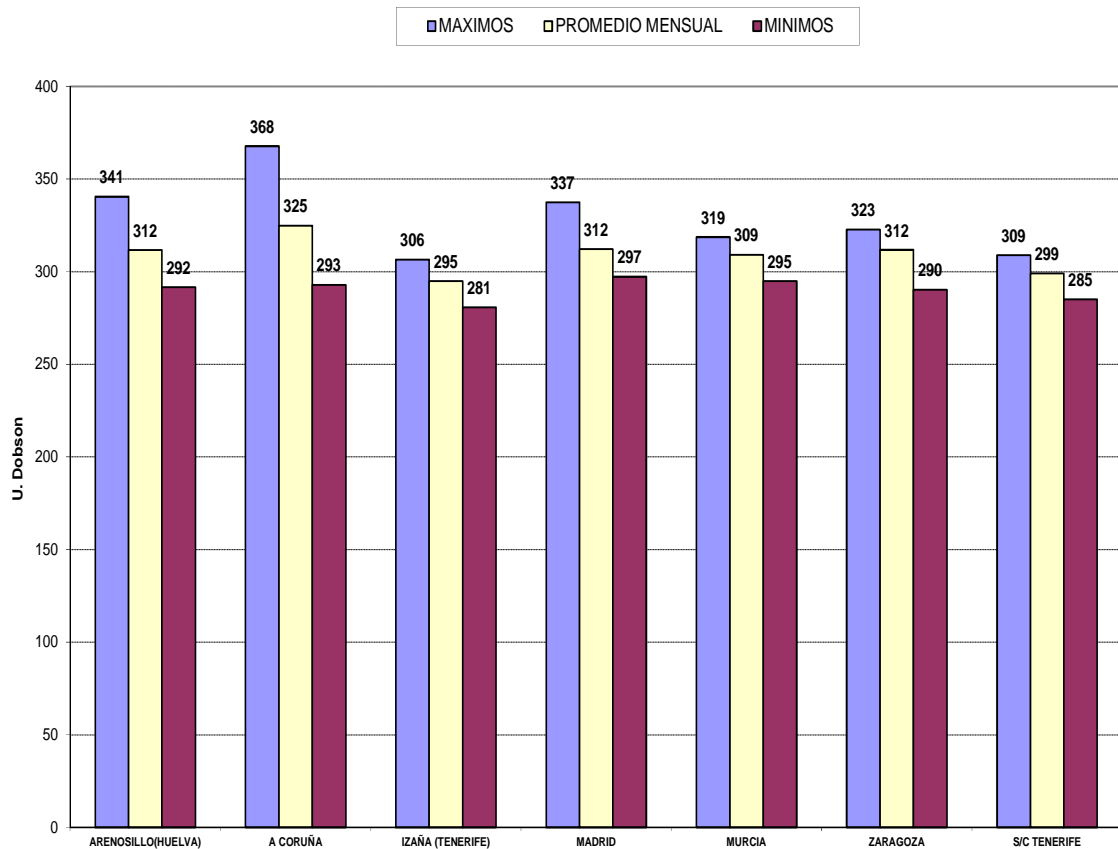
DATOS MENSUALES DE OZONO EN COLUMNA - JULIO 2015
