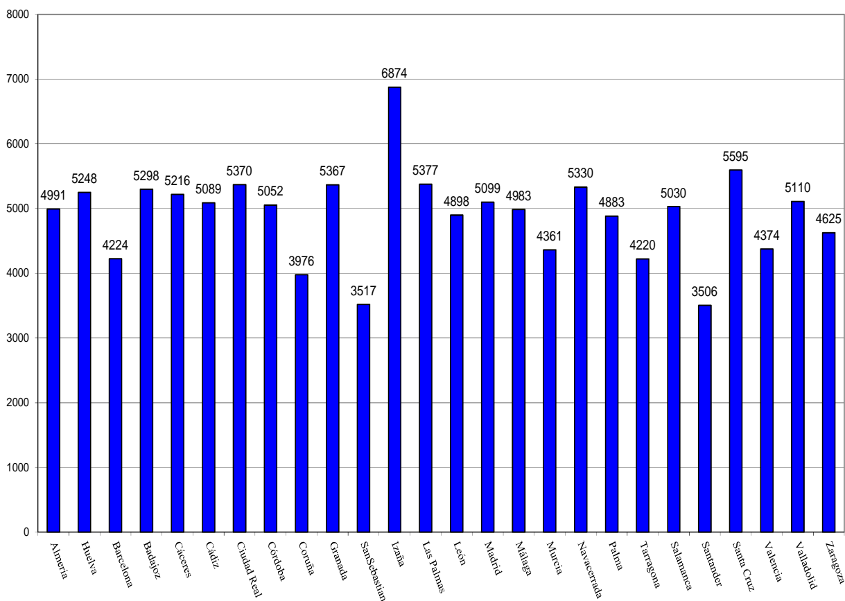
VALORES MEDIO DIARIOS DE LA RADIACIÓN UV-B EN DISTINTAS ESTACIONES DE LA RED JULIO-2015 (J/m 2 )
