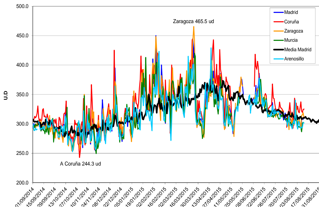
OZONO TOTAL EN COLUMNA - AÑO AGRÍCOLA 2014-2015
