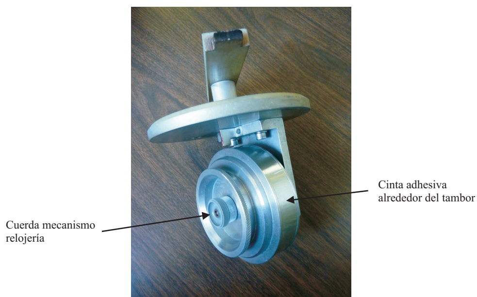
Lámina 3 b. Cabezal extraíble del captador Hirst, con tambor de muestreo.
