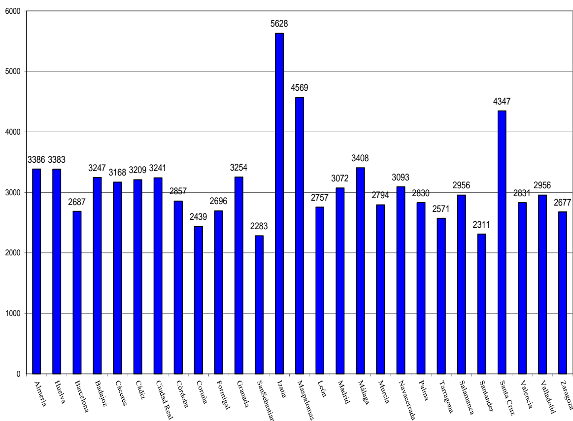
VALORES MEDIO DIARIOS DE RADIACIÓN UV Eritemática EN DISTINTAS ESTACIONES DE LA RED SEPTIEMBRE-2016 ( J/m^2 )
