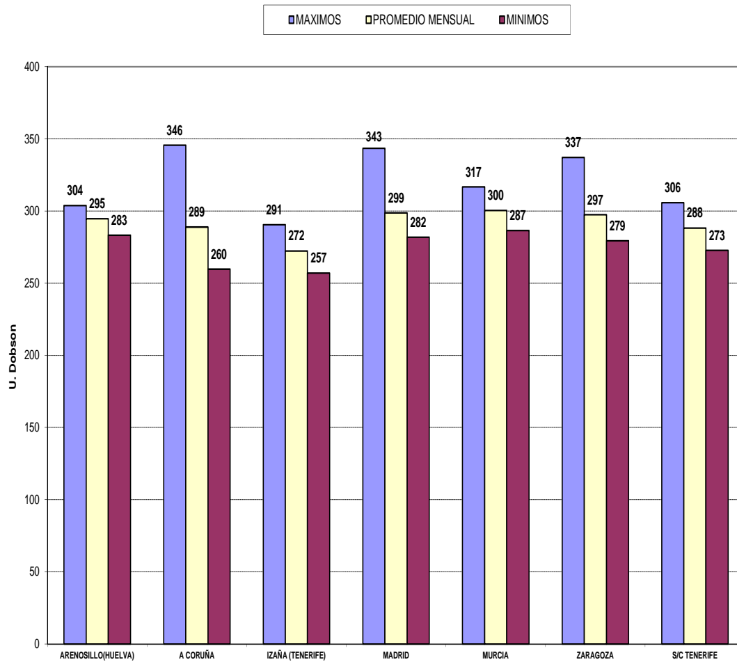
DATOS MENSUALES DE OZONO EN COLUMNA - SEPTIEMBRE 2016
