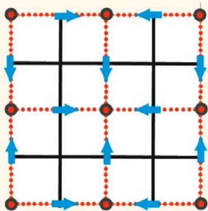
Quasi-3D MMF
