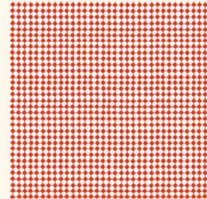
GCRM
