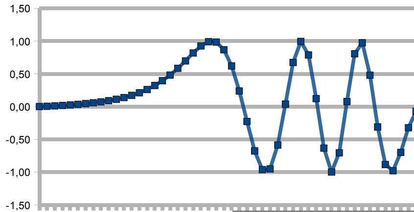
SIN( 6 PI x )
