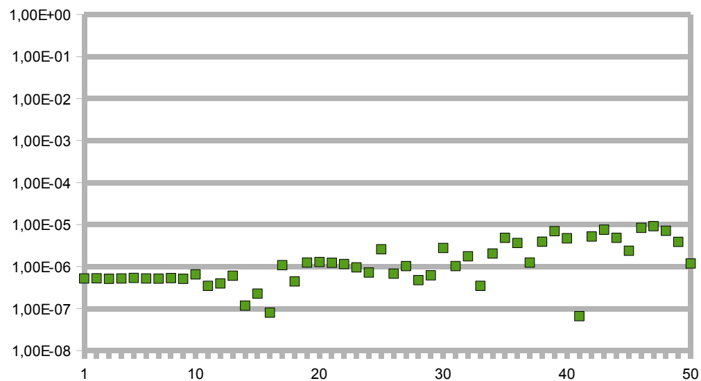
ERROR ABS D1 SIN( 6 PI x )
