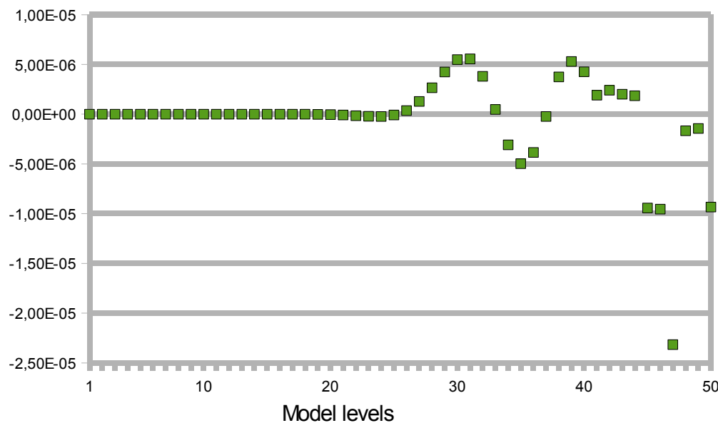
ERROR I0 SIN( 6 PI x )
