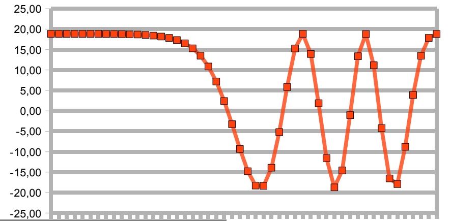
ERROR ABS D1 SIN( 6 PI x )
