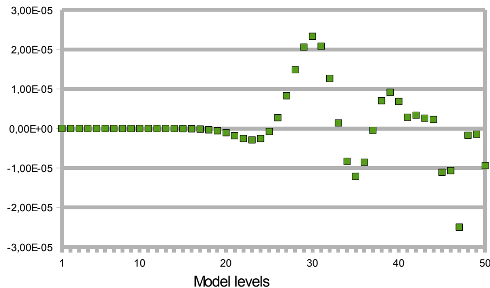
ERROR S SIN( 6 PI x )
