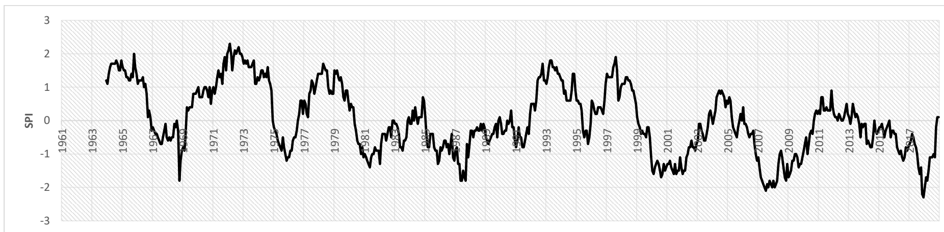
Figura. 10 Valores del SPI 36 meses en la cuenca del Pirineo oriental en el periodo 1961-2018
