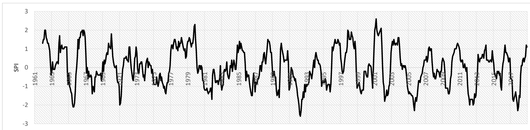
Figura. 12 Valores del SPI_{12 \text{ meses}} en la cuenca del Duero en el periodo 1961-2018
