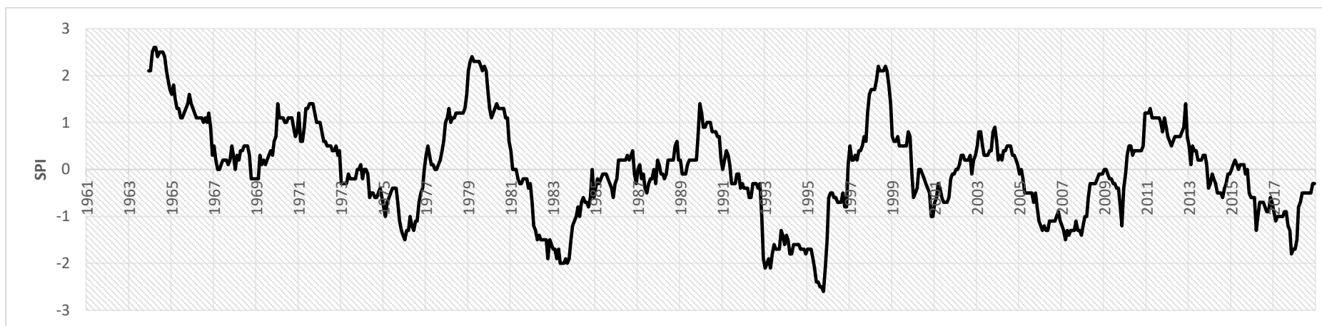
Figura. 4 Valores del SPI 36 meses en la cuenca del Guadiana en el periodo 1961-2018
