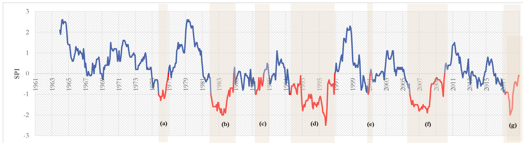
Figura. 9 Valores del SPI 36meses calculado a partir de la serie de precipitaciones mensuales (1961-2018) promediadas para España peninsular, con identificación de periodos de sequía mediante letras y colores en rojo.
