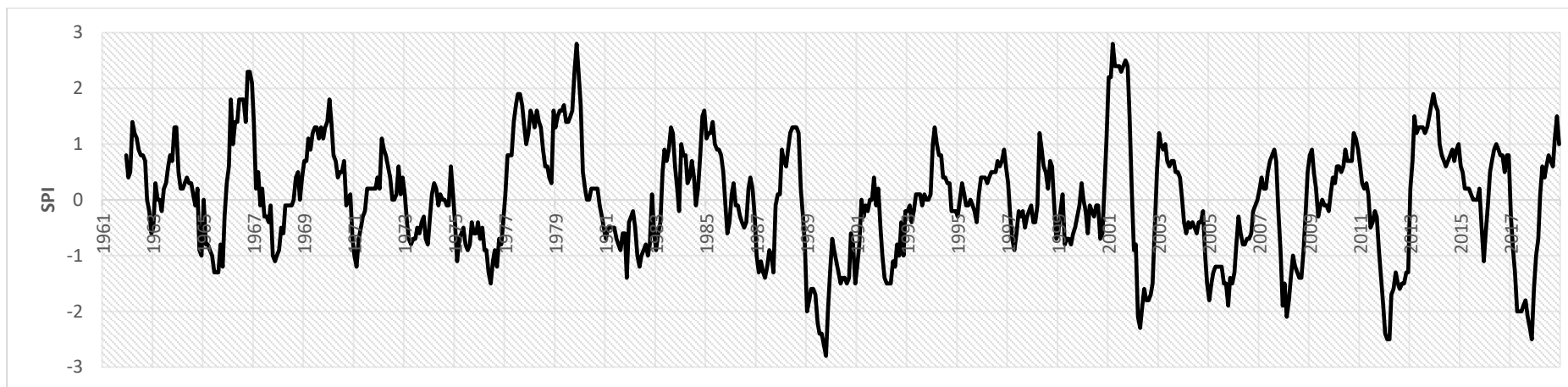
Figura. 11 Valores del SPI_{12 \text{ meses}} en la cuenca del Norte y Noroeste en el periodo 1961-2018
