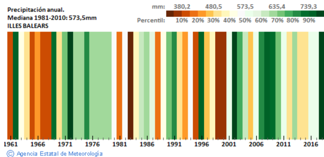
Figura. 35 Precipitación anual en la Comunidad Autónoma de illes Balears en función de su respectivo percentil.
