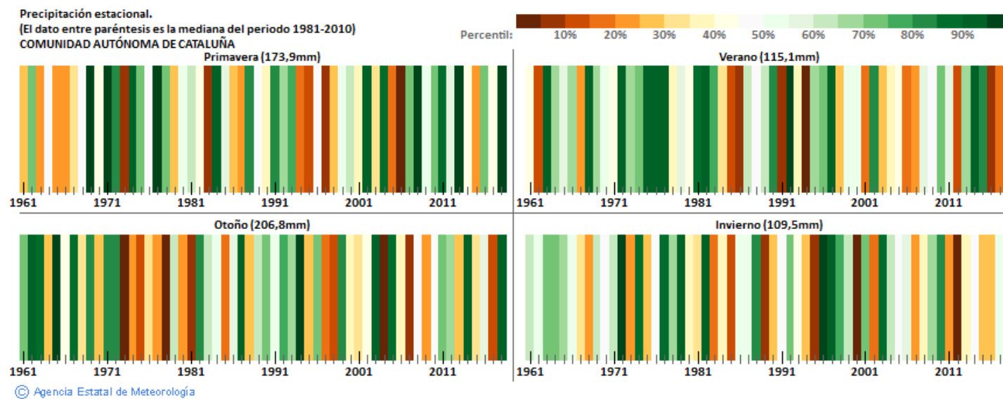
Figura. 18 Precipitación estacional en la Comunidad Autónoma de Cataluña en función de su respectivo percentil.
