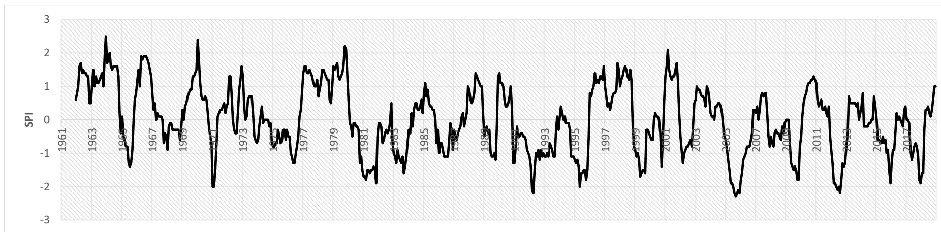
Figura. 13 Valores del SPI 12 meses en la cuenca del Tago en el periodo 1961-2018
