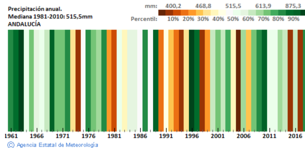
Figura. 2 Precipitación anual en la Comunidad Autónoma de Andalucía en función de su respectivo percentil.
