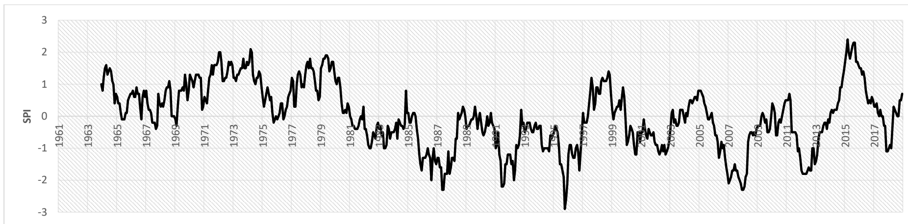
Figura. 9 Valores del SPI 36 meses en la cuenca del Ebro en el periodo 1961-2018.
