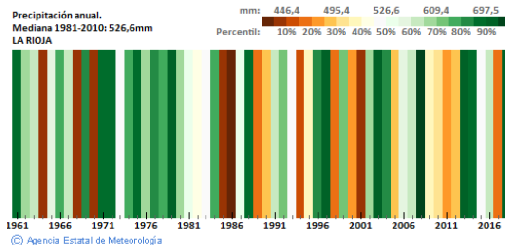
Figura. 41 Precipitación anual en la Comunidad Autónoma de La Rioja en función de su respectivo percentil.
