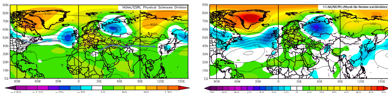
Promedios de la altura del geopotencial y anomalías para el verano de 2019. Izquierda: 300 hPa; derecha: 850 hPa. Fuente NOAA/ESRL.
