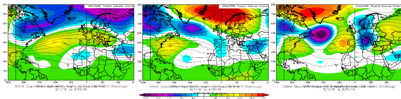
Valor y anomalía medios de la altura del geopotencial en 300 hPa para los meses de marzo, abril y mayo de 2019. Fuente NOAA/ESRL.
