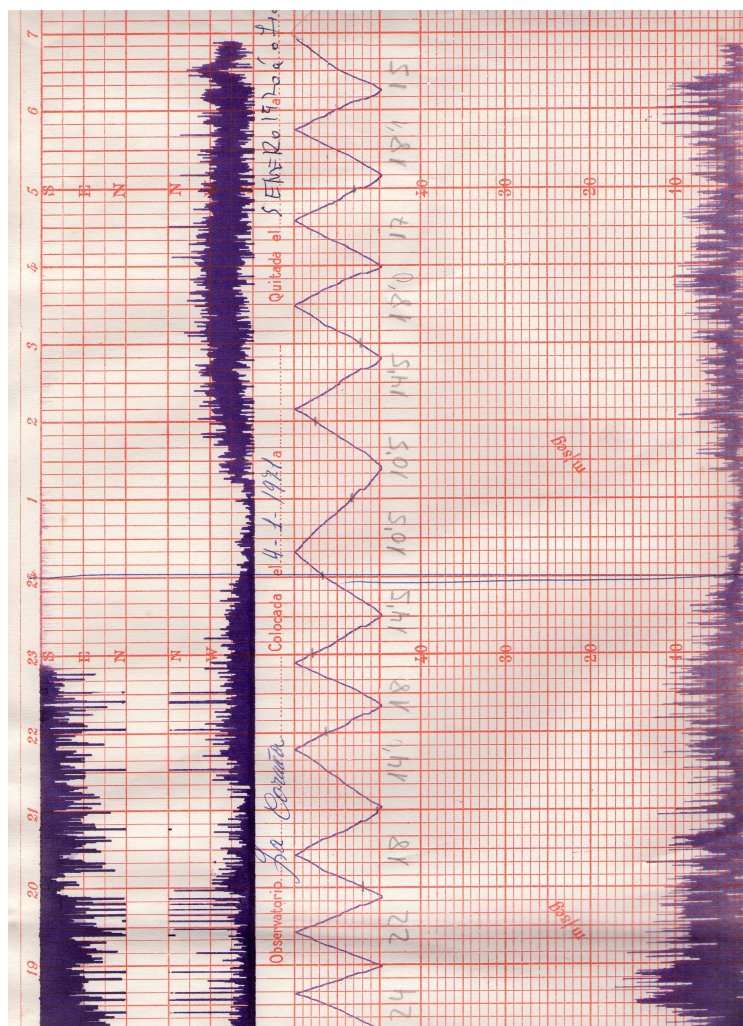
Figura 5.0.1. Banda de anemocinógrafo. A Coruña, 4 de enero de 1971, con registros de dirección, recorrido y velocidad del viento.
