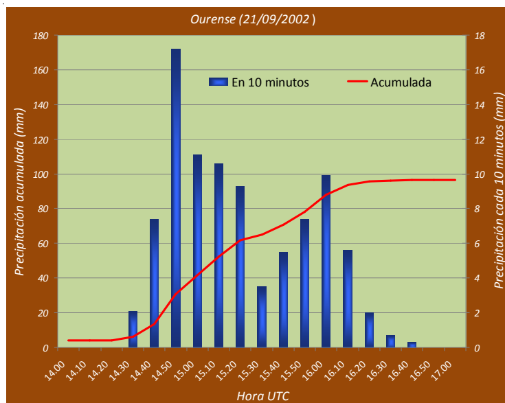
Figura 4.3.2. Precipitación recogida en el observatorio de Ourense durante la tarde del día 21 de septiembre de 2002.
