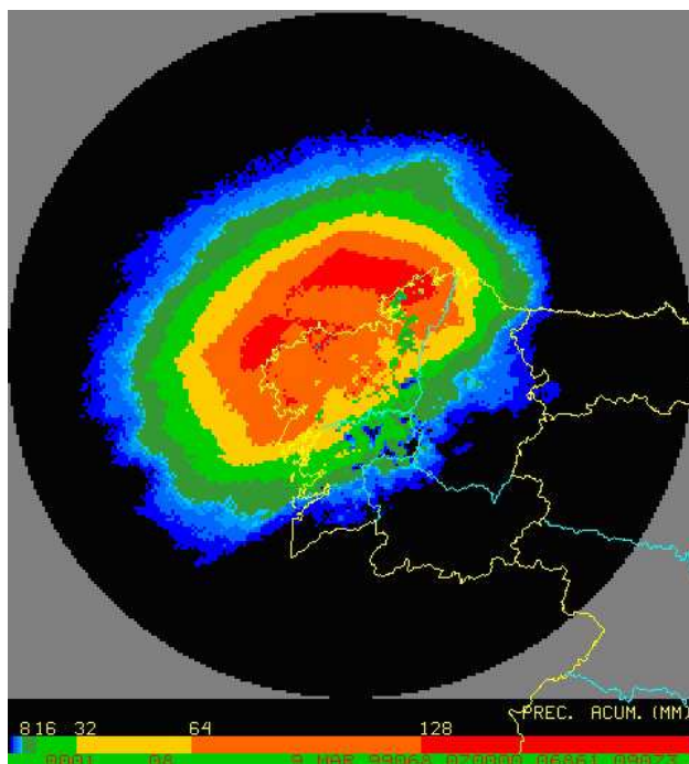
Figura 9.2.2. Acumulación de precipitación estimada por el radar de AEMET en Galicia entre las 07 horas UTC del día 8 de marzo de 1999 y la misma hora del día 9. Este periodo fue extremadamente lluvioso en el noroeste de Galicia. En particular el observatorio de A Coruña registró la máxima precipitación en 24 horas de su larga serie de observaciones: 132,7 mm.
