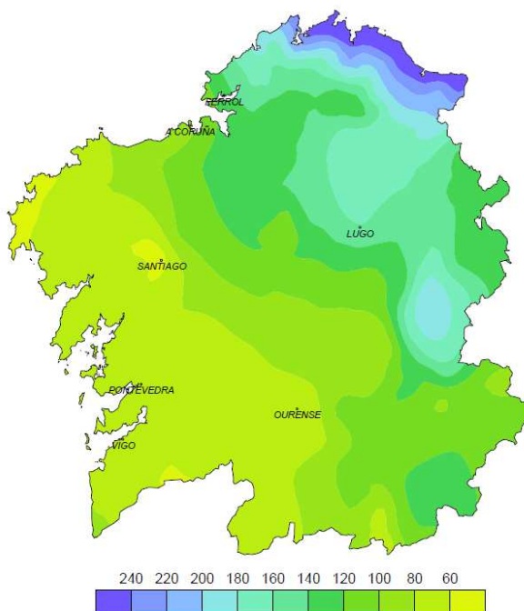
Figura 9.1.2. Mapa de precipitación total mensual en Galicia durante el mes de junio de 2010. Puede verse el gradiente de lluvia en dirección suroeste-nordeste y la acumulación de precipitación en la costa de Lugo. La escala está graduada en mm.
