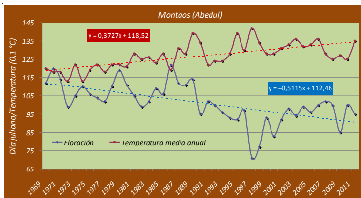
Figura 8.2.1. Evolución de la fecha de floración del abetul y de la temperatura media anual (décimas de °C) en la estación de Montaos.
