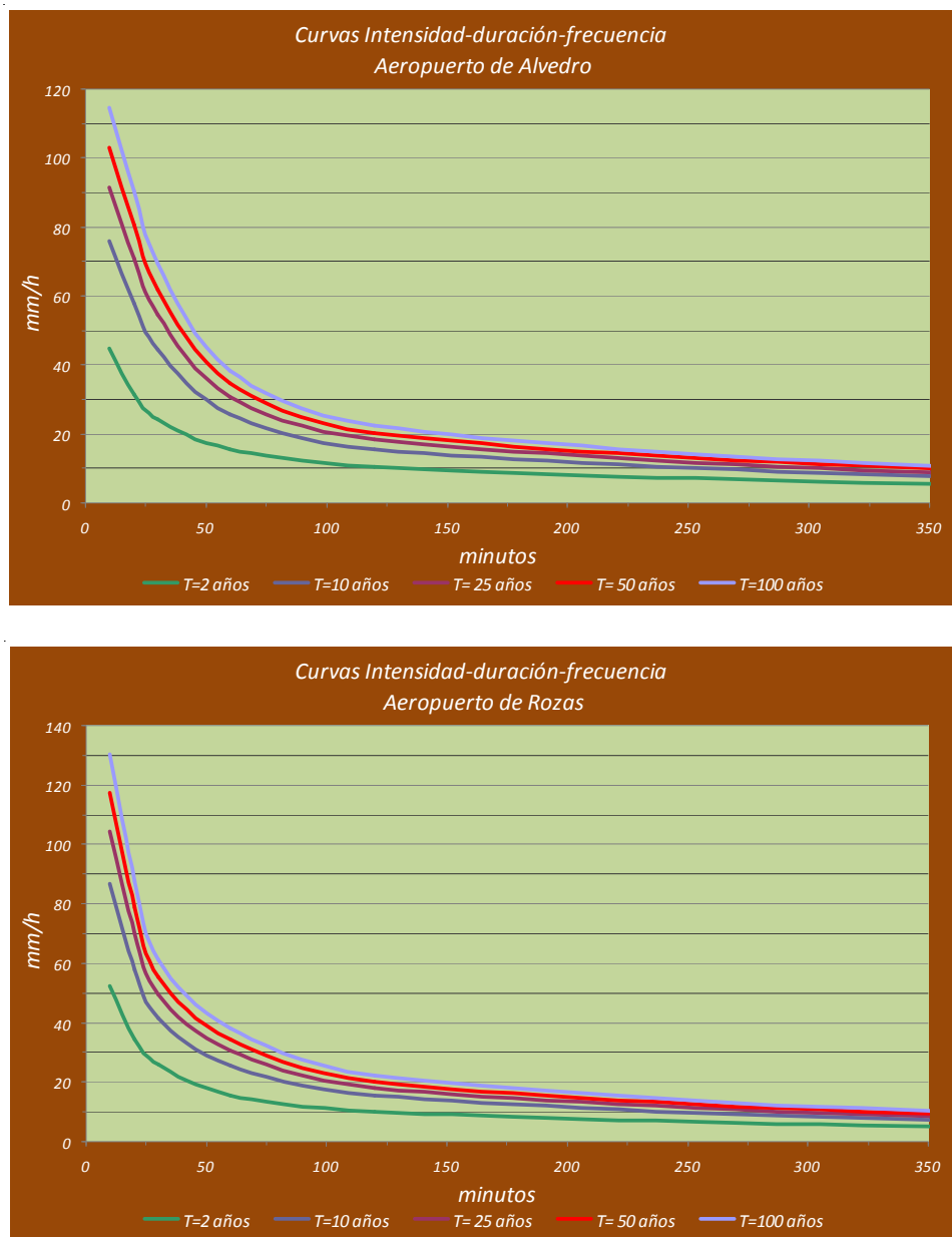
Figura 4.2.1. Curvas de intensidad-duración-frecuencia para los observatorios del aeropuerto de Alvedro (arriba) y del aeródromo de Rozas (abajo). Los cálculos de los periodos de retorno se efectuaron mediante el ajuste a la distribución de Gumbel.
