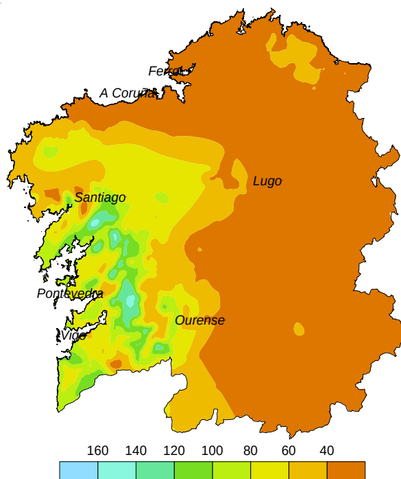
Figura 9.4.2. Precipitación acumulada el día 13 de diciembre de 2012 (imagen superior) en mm y estimación de la precipitación acumulada mediante medidas de radar (la escala inferior está también graduada en mm). Se observa una clara subestimación por parte del radar de la lluvia recogida en la zona suroccidental de Galicia. En particular en la estación de Rois.
