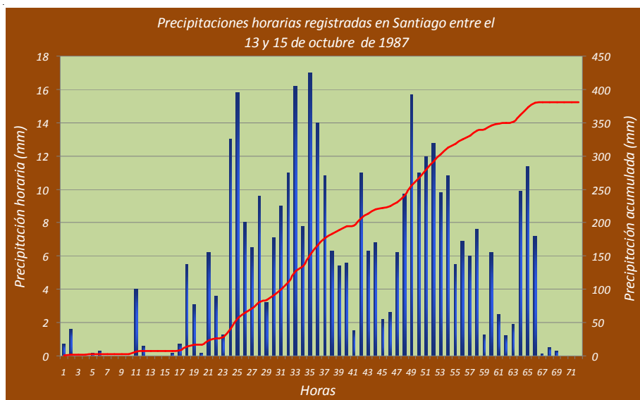
Figura 9.8.2. Valores horarios y acumulados del episodio de precipitación registrado en el aeropuerto de Santiago entre el 13 y el 15 de octubre de 1987.
