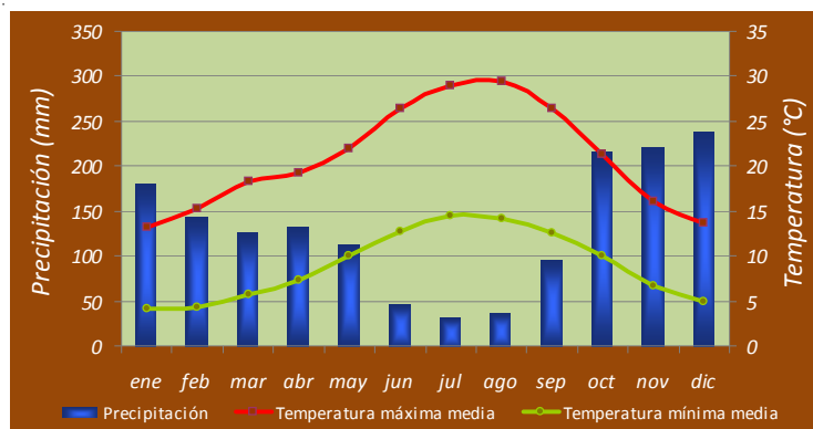
Figura 9.6.1. Valores medios mensuales de precipitación y temperaturas extremas en la estación de Ponteareas. Periodo 1971-2000.
