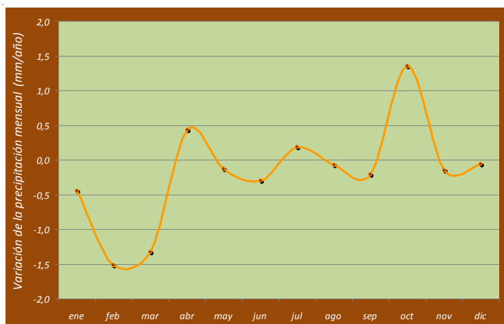
Figura 4.4.3. Tendencia media anual (mm/año) de la precipitación para cada mes del año en Galicia desde 1950 hasta 2012.
