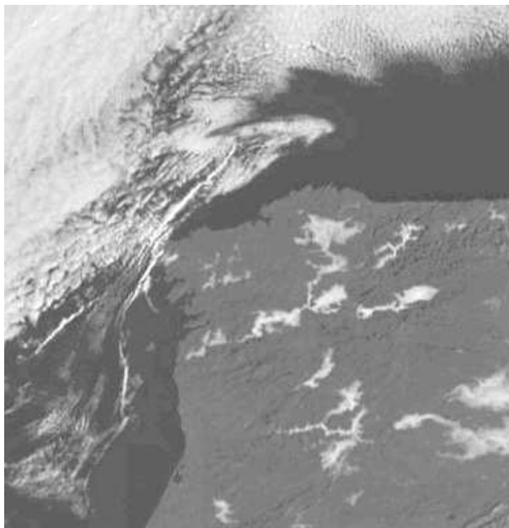
Figura 9.7.2. Imagen visible del satélite Meteosat correspondiente a las 9.30 horas del 25 de enero de 2012. Se observan con claridad las nieblas siguiendo, entre otros, los cursos del Miño, del Sil y del Navia. Hay una mancha más extensa en el entorno de Vilalba.
