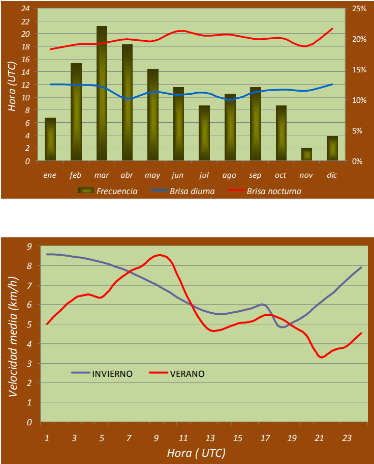
Figura 5.3.6. Brisa observada en la estación de Padrón (A Coruña). Frecuencia mensual junto con las horas promedio de inicio y final en el gráfico superior. Velocidad media de la brisa en invierno y verano a lo largo del día en la gráfica inferior.
