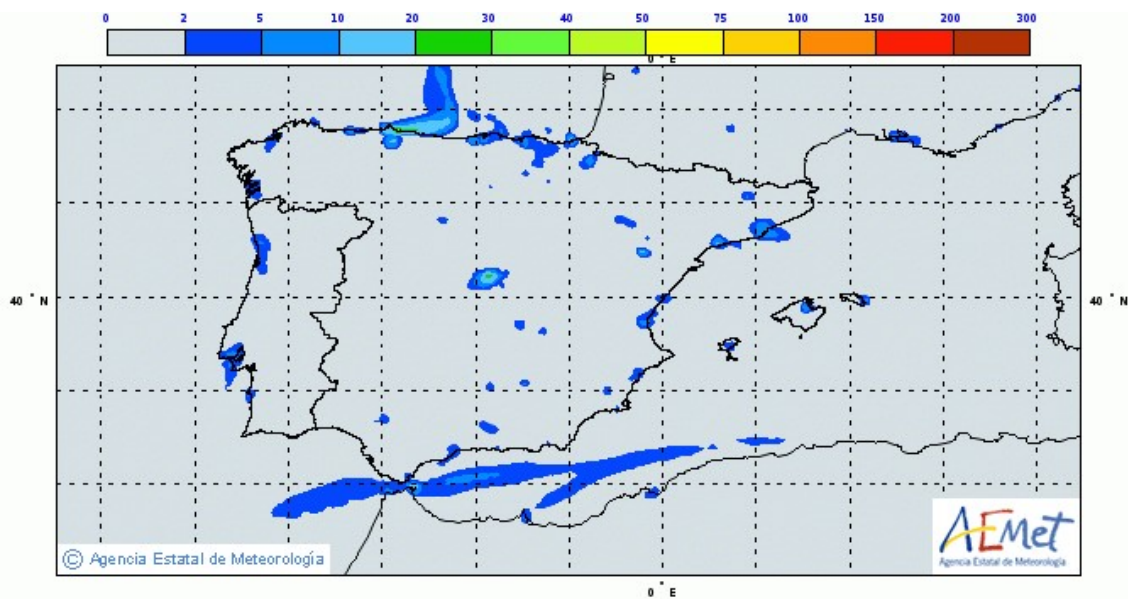
Fig. 2 – Concentraciones previstas en superficie de NO ( \mu\text{g}/\text{m}^3 ) generados por MOCAGE en el dominio Regional para el día 14 de agosto de 2019 a las 12 horas UTC.
