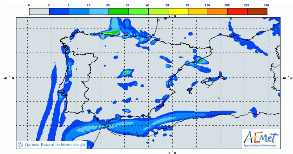
Fig. 1 – Concentraciones previstas en superficie de NO 2 (µg/m 3 ) generados por MOCAGE en el dominio Regional para el día 14 de agosto de 2019 a las 12 horas UTC.
