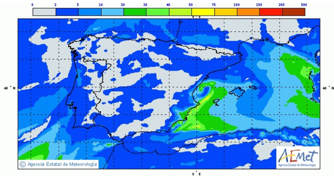
Fig. 7 – Concentraciones previstas en superficie de PM2.5 ( \mu\text{g}/\text{m}^3 ) generados por MOCAGE en el dominio Regional para el día 14 de agosto de 2019 a las 12 horas UTC.
