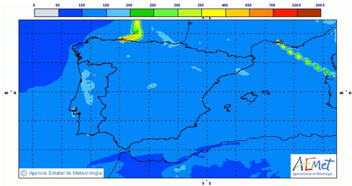
Fig. 5 – Concentraciones previstas en superficie de CO (µg/m 3 ) generados por MOCAGE en el dominio Regional para el día 14 de agosto de 2019 a las 12 horas UTC.
