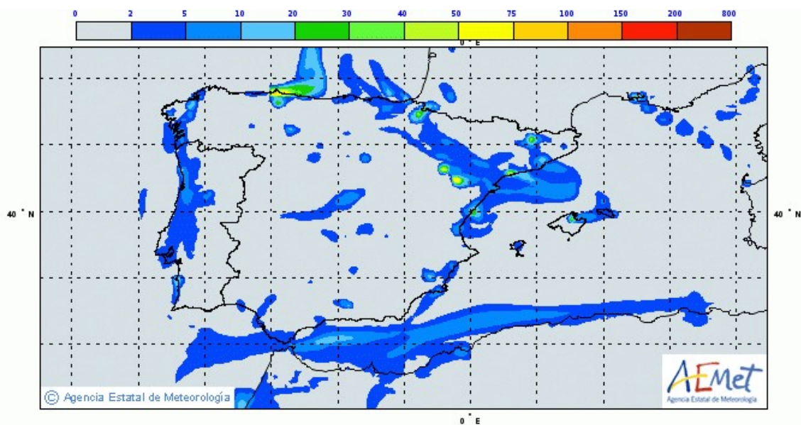
Fig. 3 – Concentraciones previstas en superficie de SO 2 ( \mu\text{g}/\text{m}^3 ) generados por MOCAGE en el dominio Regional para el día 14 de agosto de 2019 a las 12 horas UTC.
