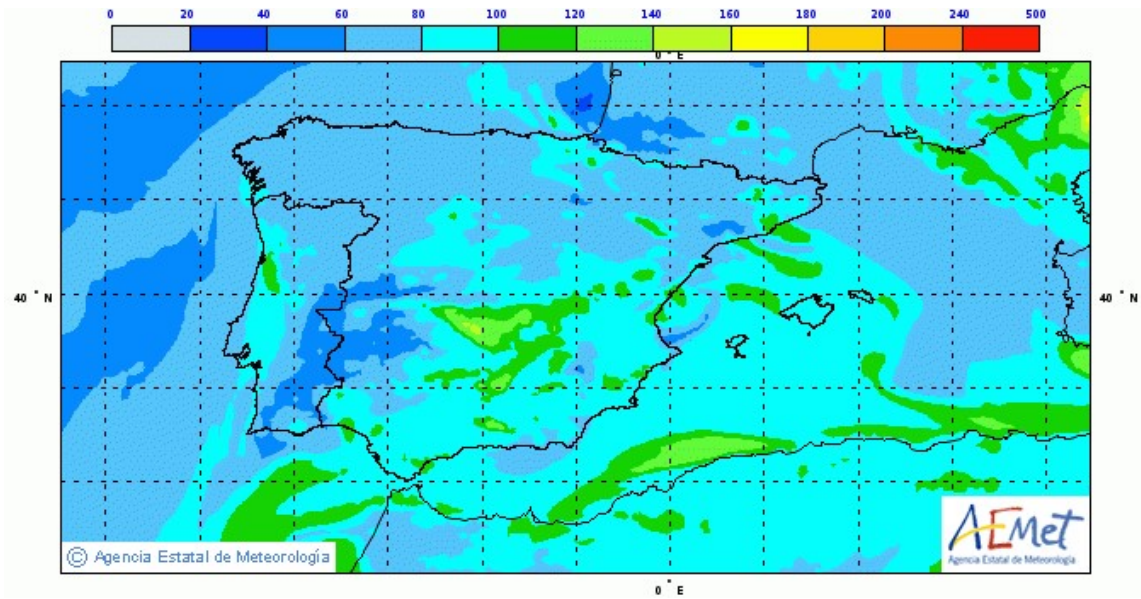
Fig. 4 – Concentraciones previstas en superficie de O 3 (µg/m 3 ) generados por MOCAGE en el dominio Regional para el día 14 de agosto de 2019 a las 12 horas UTC.
