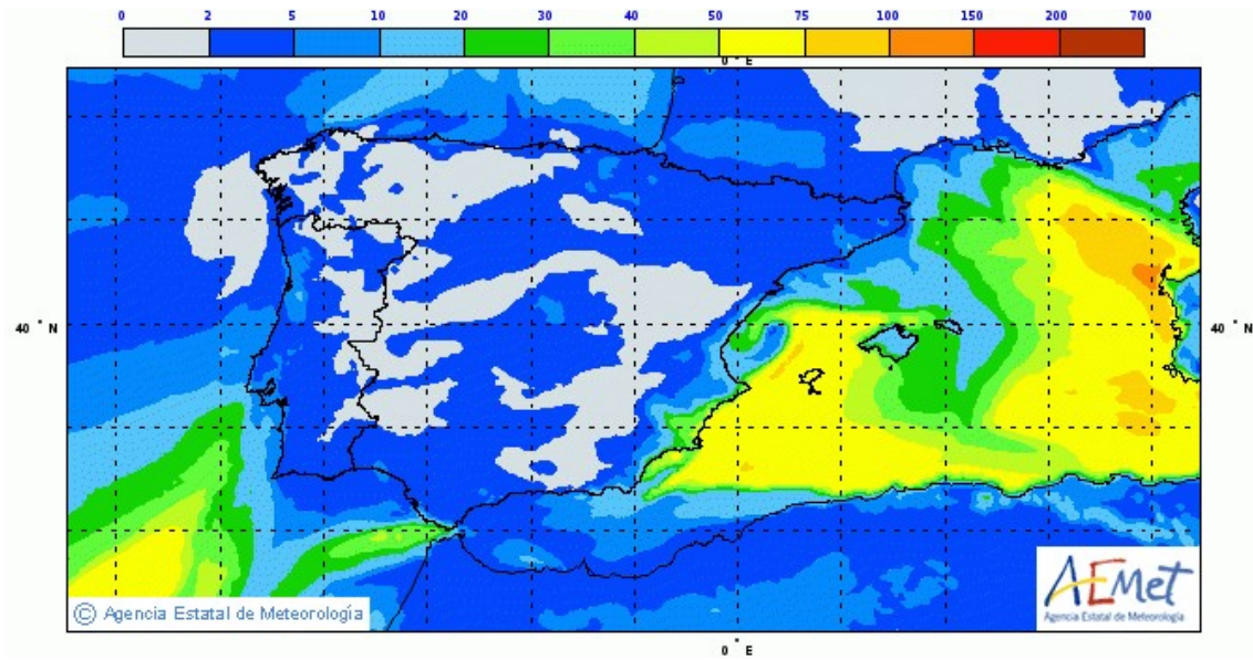
Fig. 6 – Concentraciones previstas en superficie de PM10 ( \mu\text{g}/\text{m}^3 ) generados por MOCAGE en el dominio Regional para el día 14 de agosto de 2019 a las 12 horas UTC.
