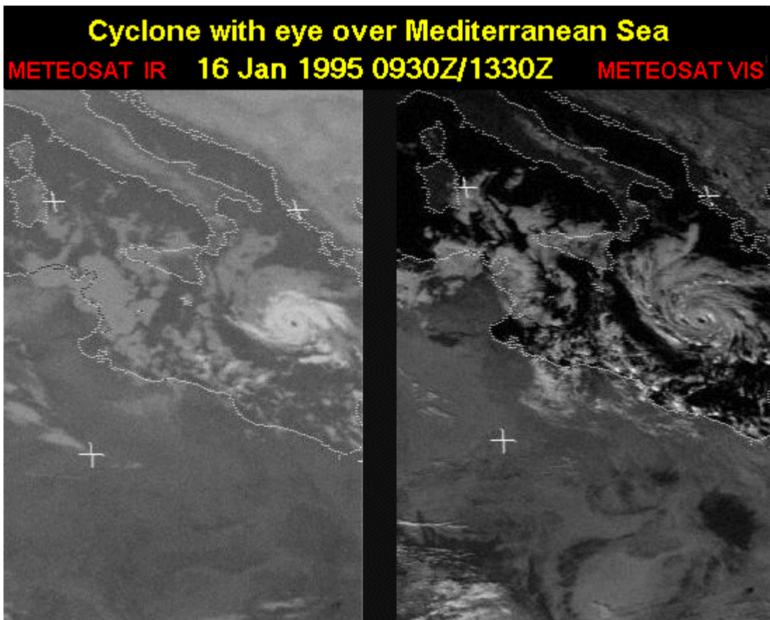
Par de imágenes de un ciclón mediterráneo observado por el Meteosat el 16 de enero de 1995. Izquierda imagen IR de las 09:30 UTC y visible, VIS, de las 13:30 UTC. Fuente: http://www.mindspring.com/~jbeven/intr0008.htm
