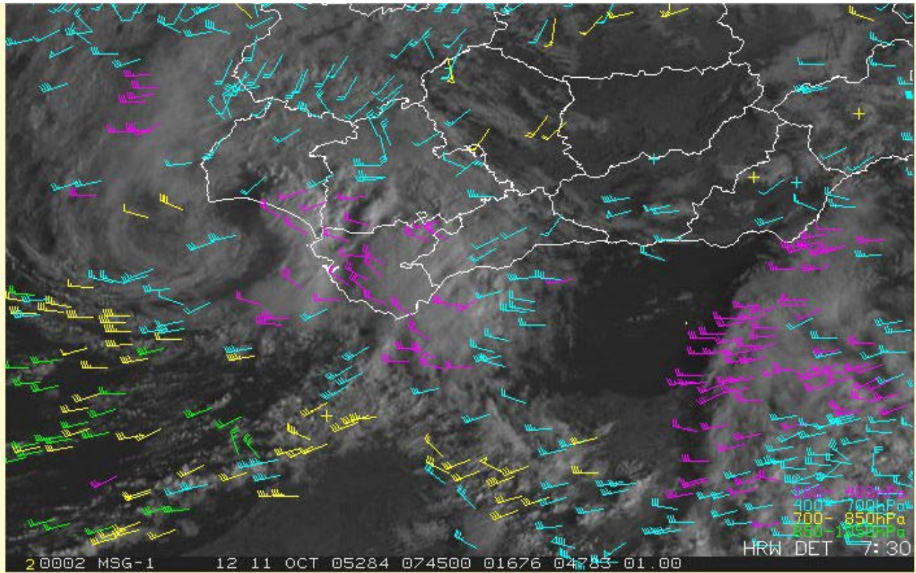
Vientos, en nudos, estimados a partir de trazadores nubosos por niveles con la imagen de fondo VIS de alta resolución del MET8, MSG-1, a las 07:45 UTC (09:45 hora oficial). Vientos estimados entre superficie y 850 hPa, en verde; resto de los vientos, según escala adjunta.
